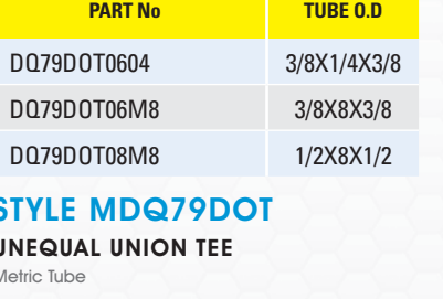
STYLE DQ79DOT UNEQUAL UNION TEE
